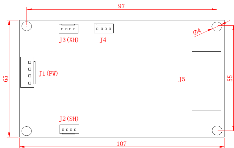
图 2.2 BL2000-HXJ-V9 尺寸图 (单位 mm)
